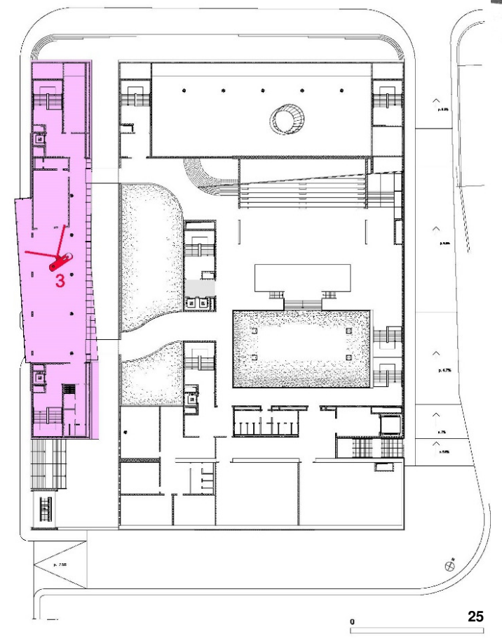
Piano secondo (mq 910)
