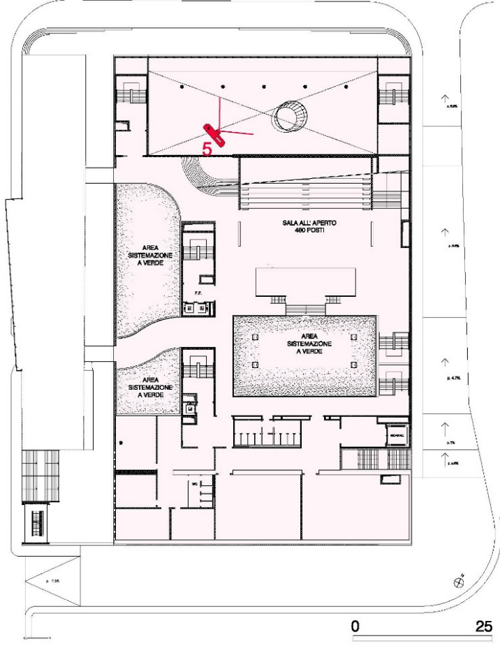
Piano secondo copertura (mq 3300) - Giardino pensile, servizi
